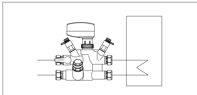
Пример: Регулирование системы только с помощью четырехходового вентилей „Cocoon 4TR“.
