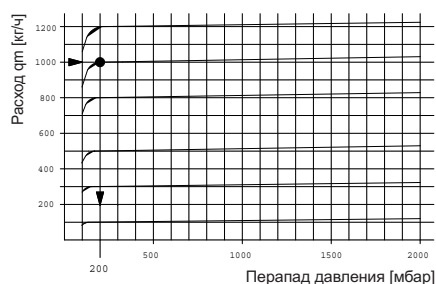
Характеристики расхода при различной преднастройке
