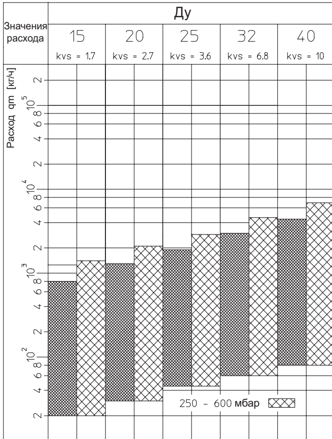
Значения расхода регулятора перепада давления „Нусоcon DTZ“ при перепаде давления в стояке 50–300 мбар или 250–600 мбар.
