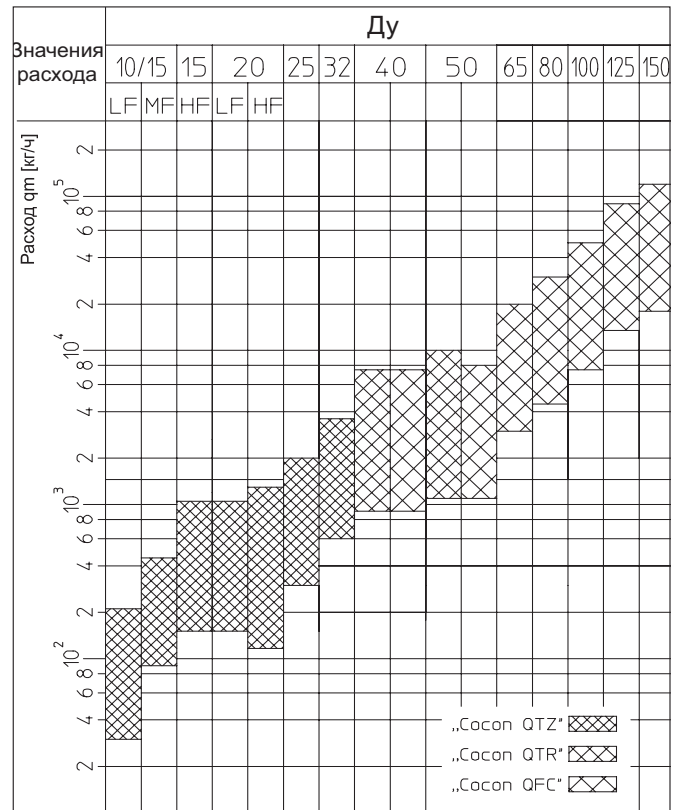
„Cosoon QTZ/QFC“ с приводами
