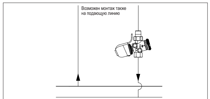
Пример: Регулирование расхода с помощью вентиля „Cosoon QTZ“.
