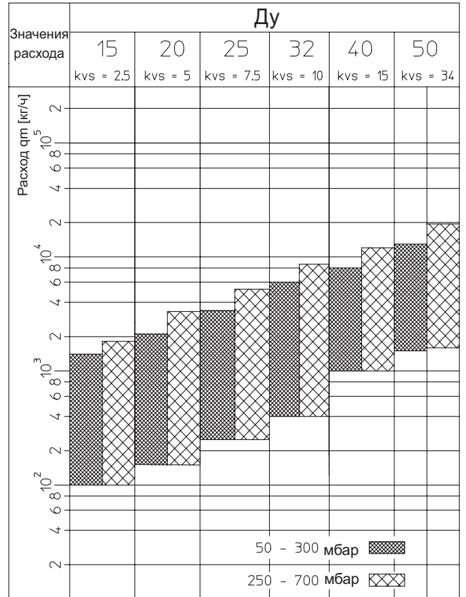
Значения расхода регулятора перепада давления „Нусоcon DTR“ при перепаде давления в стояке 50–300 мбар или 250–700 мбар.
