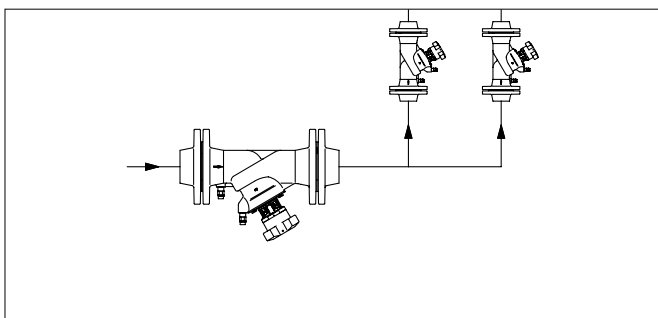
Пример: Система отопления с фланцевыми регулирующими вентилем.
