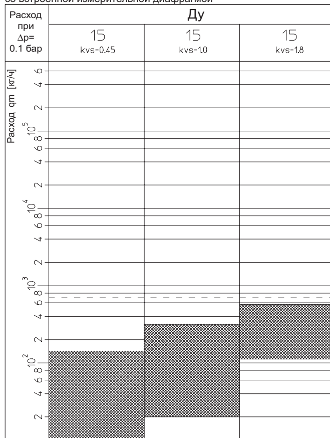
Четырехходовой регулирующий вентиль „Cocoon 4TR“ со встроенной измерительной диафрагмой
