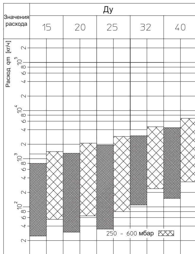
Значения расхода регулятора перепада давления „Нусоcon DTZ“ при перепаде давления в стояке 50–300 мбар или 250–600 мбар и ограничение расхода на регулирующем вентиле „Нусоcon VTZ“.
