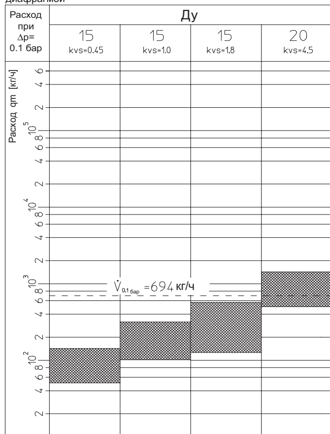
Регулирующий вентиль „Cocoon 2TZ“ со встроенной измерительной диафрагмой
