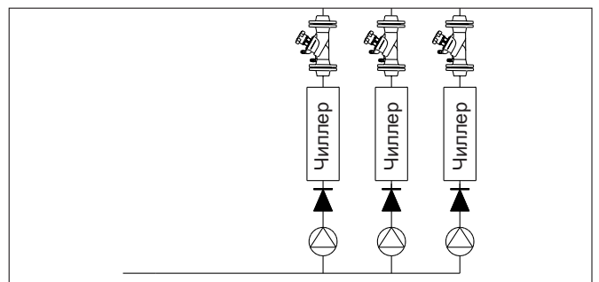
Пример: Система охлаждения с фланцевыми регулирующими вентилем.
