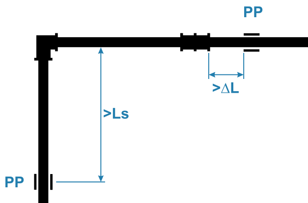
Правильное расположение подвижных опор.
